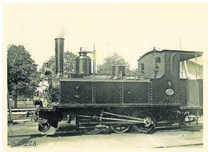
La loco No 5 du LEB a été construite en 1890. DR
